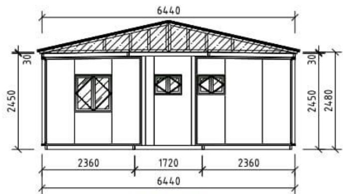
30尺北立面图
