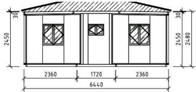
30尺南立面图
