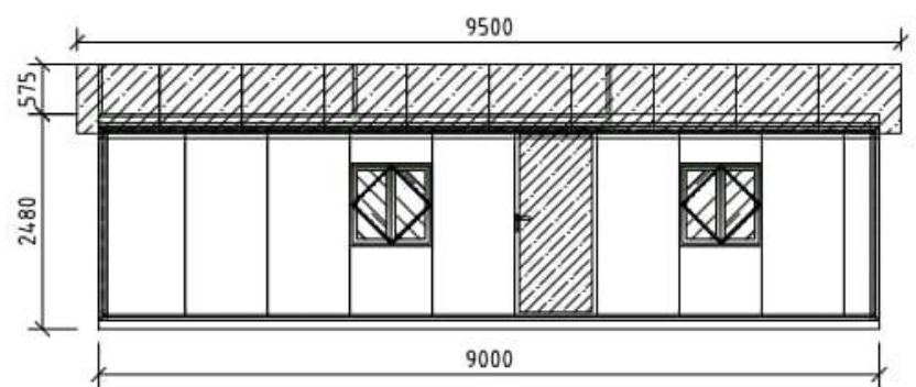
30尺西立面图
